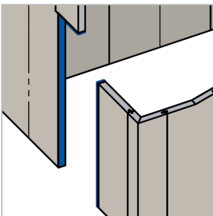
FIX-PRO-MAK 80 mm, sur le pourtour des 3 côtés de la baie de porte
