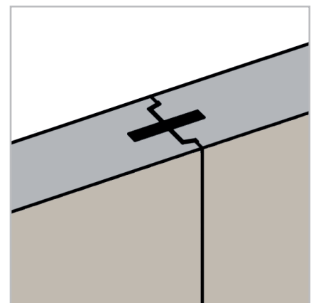
Jonction des panneaux par languette et fraisage en V
