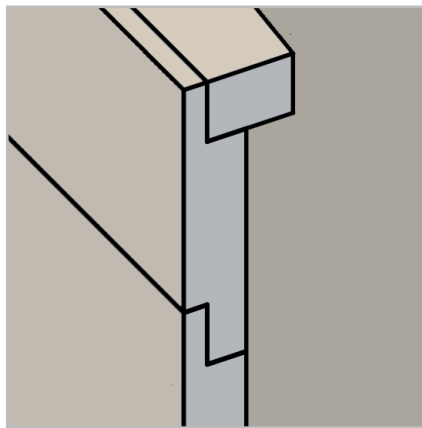
Relèvement des parois et support de toit avec chants décalés
