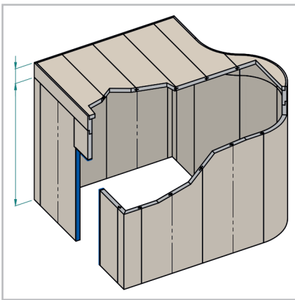
Hauteur de paroi flexible, possibilité de parois plus hautes par relèvement des parois
